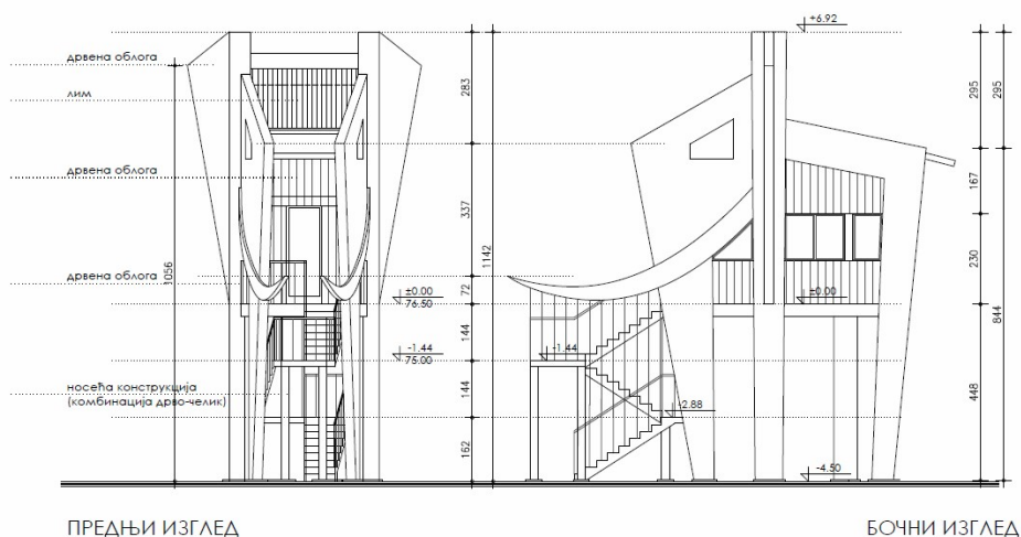
ПРЕДЊИ И БОЧНИ ИЗГЛЕД р 1:75
